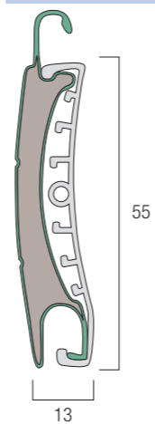
Profilo Duero 55
